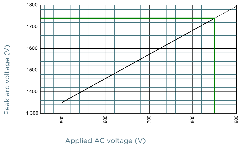
Size 73 aR 850V
