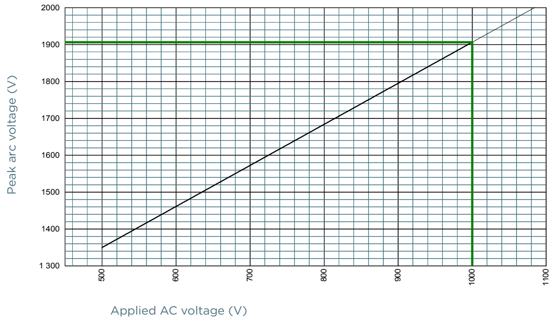
Size 73 aR 1100V
