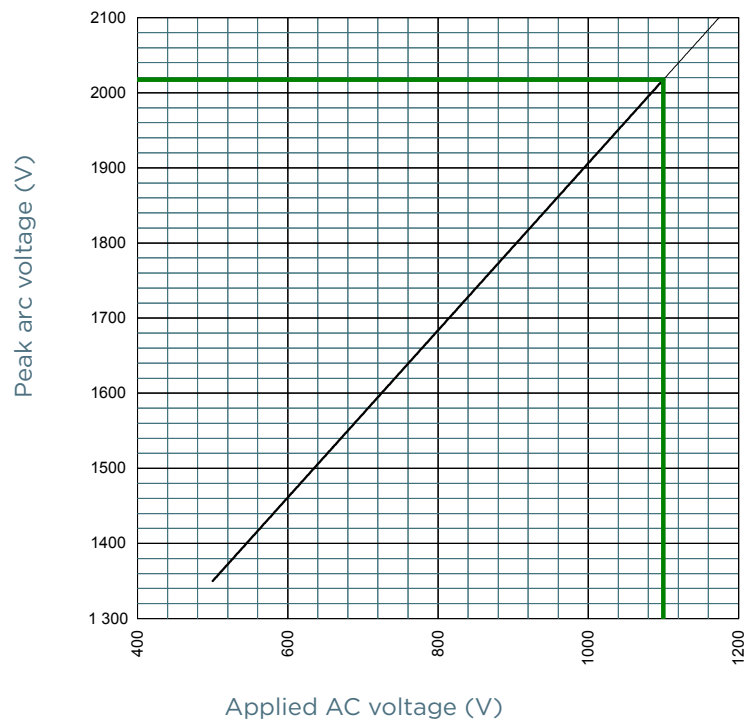
Size 73 aR 1100V
