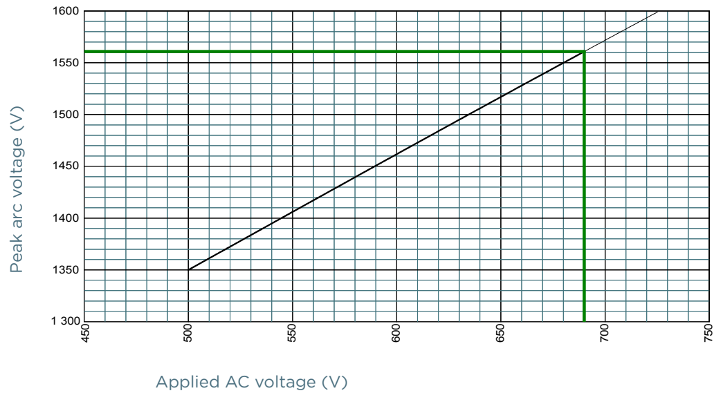
Size 73 aR 850V
